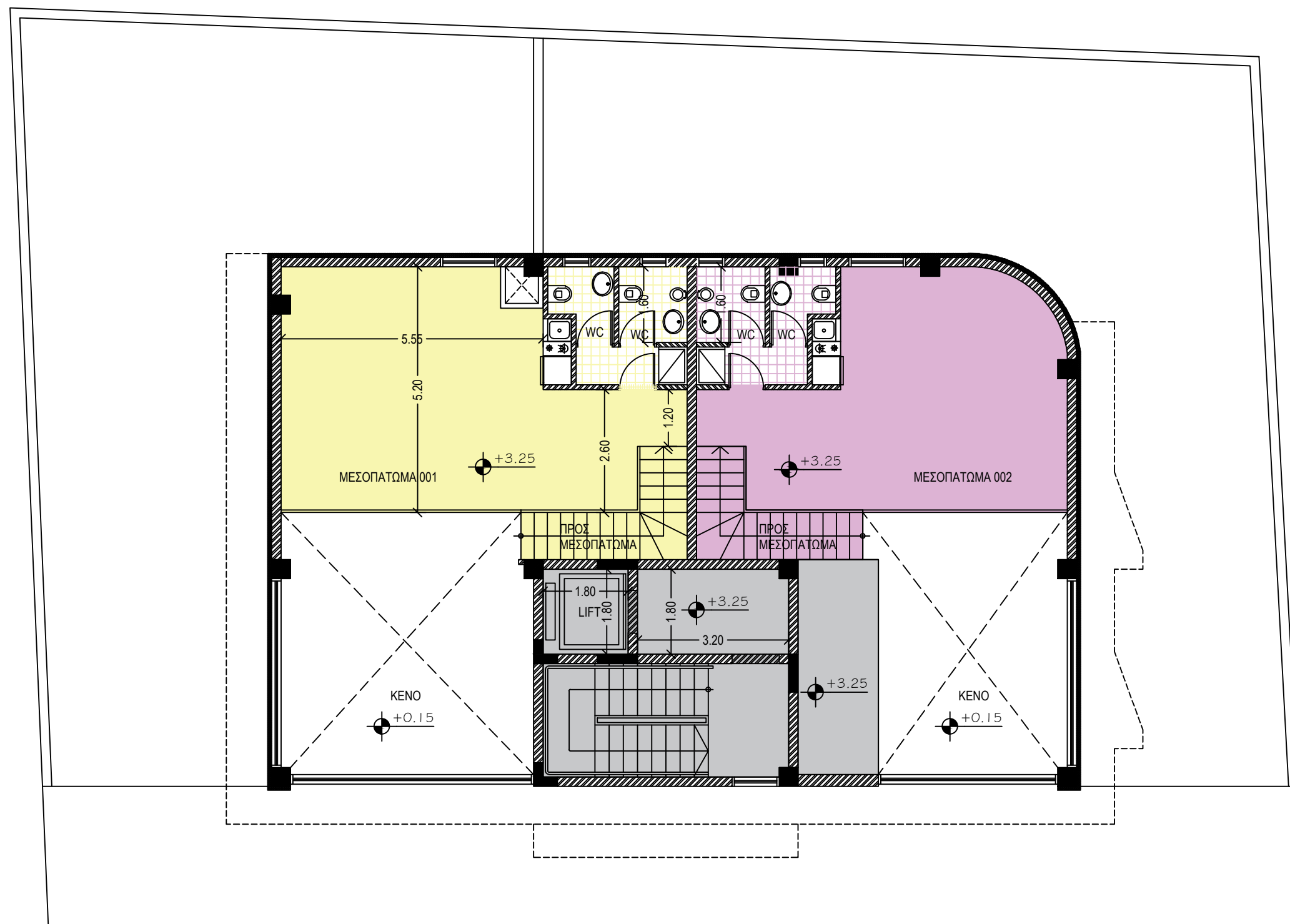
ΚΑΤΟΨΗ ΜΕΣΟΠΑΤΩΜΑΤΟΣ
