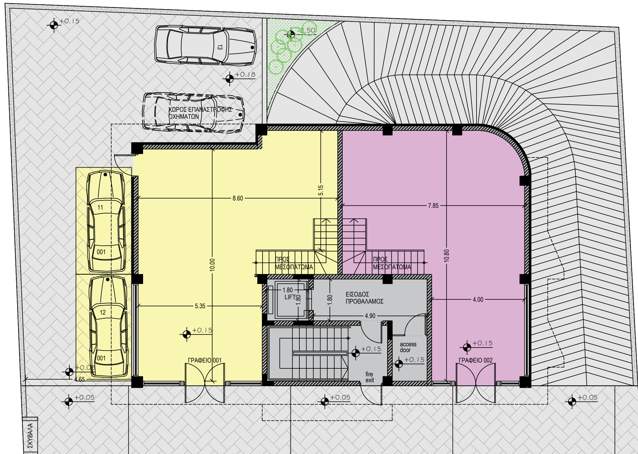
ΚΑΤΟΨΗ ΙΣΟΓΕΙΟΥ
